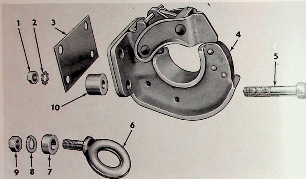
FIG. 65—PINTLE HOOK
